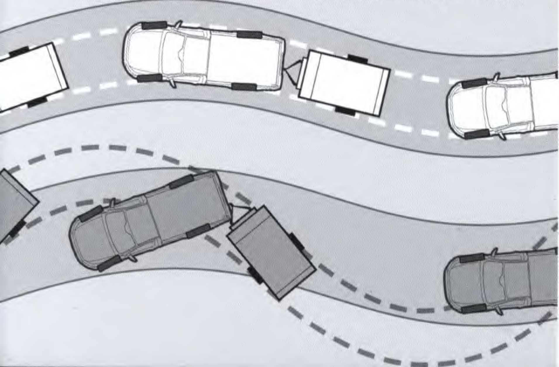
ระบบควบคุมการทรงตัวขณะลากจูง (Trailer Sway Control)
