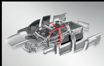
โครงสร้างตัวถังนิรภัย FSF (FULL SPACE FRAME)
