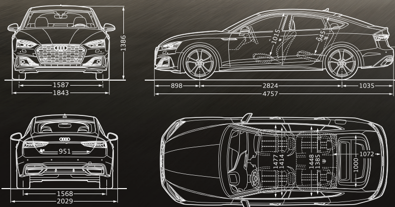
ขนาดและมิติ หน่วย: มิลลิเมตร
